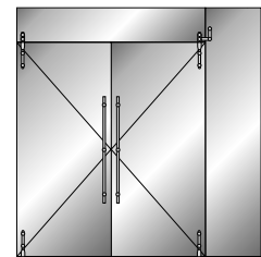
Door type 21 + 1xSET 2 + 1xSET 3
